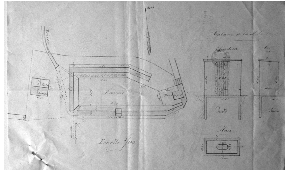
Plans du lavoir Saint-Délo (Archives municipales de Plovévet)
